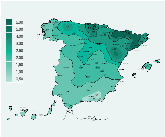
Mapa de densidad de impactos sobre el terreno (Ng). Ng: densidad de impacto/km 2 y año. Fuente: Código Técnico Edificación (CTE) – SU8 (Seguridad frente al rayo).
