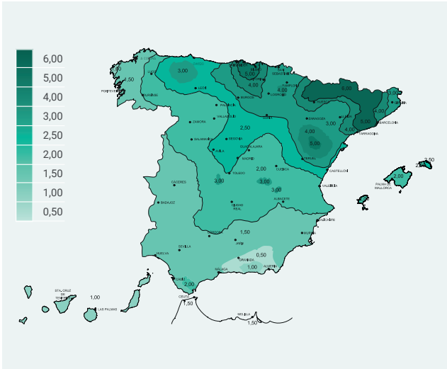
Mapa de densidad de impactos sobre el terreno (Ng). Ng: densidad de impacto/km² y año. Fuente: Código Técnico Edificación (CTE) – SU8 (Seguridad frente al rayo).
